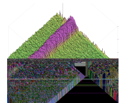
3D-Bild einer Schweißnahtvermessung
